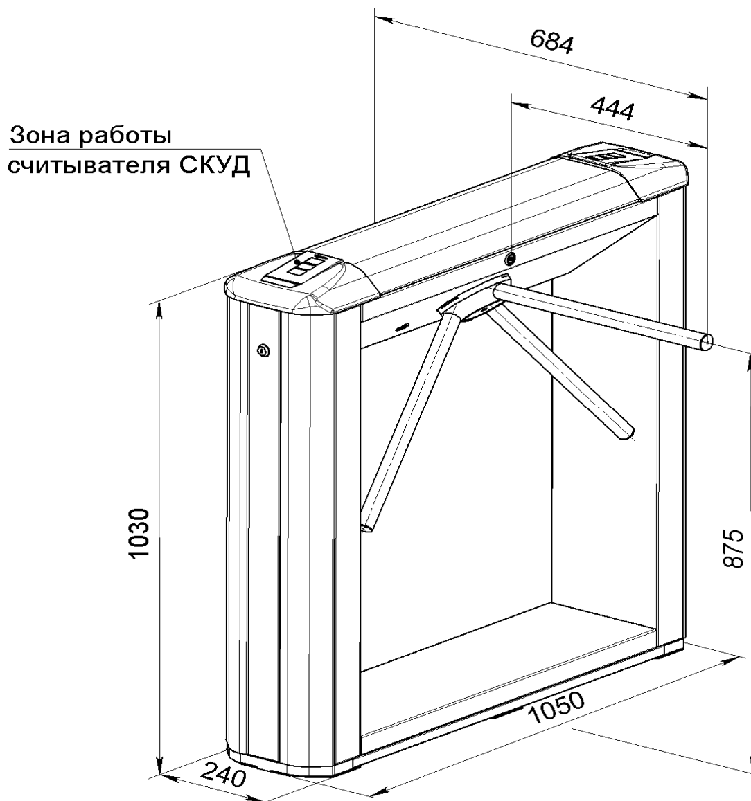
Рисунок 2 — Габаритные размеры KTC01.3
