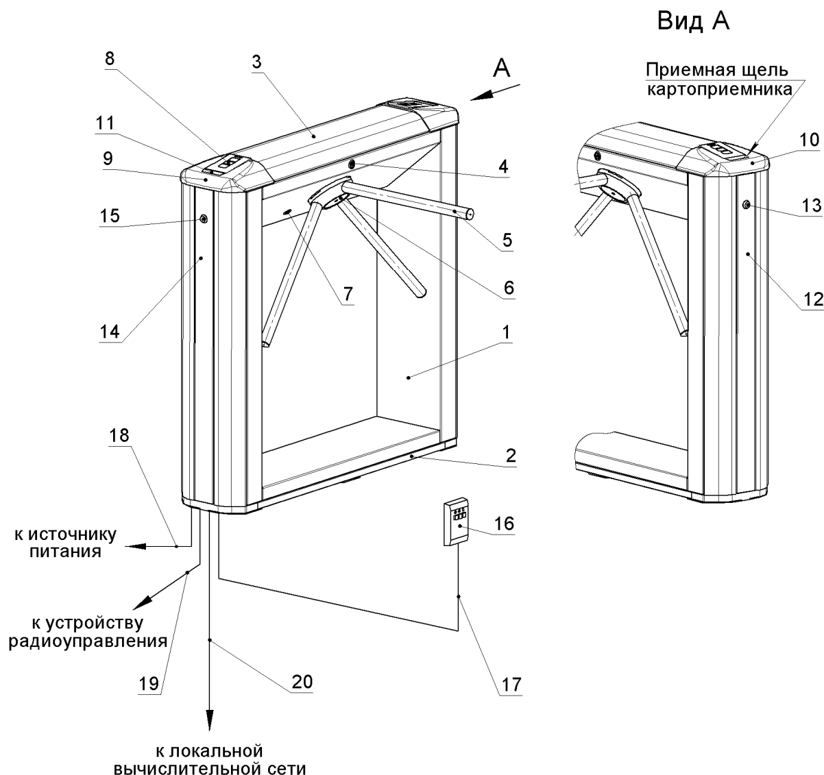
Рисунок 1 — Устройство KTC01.3
