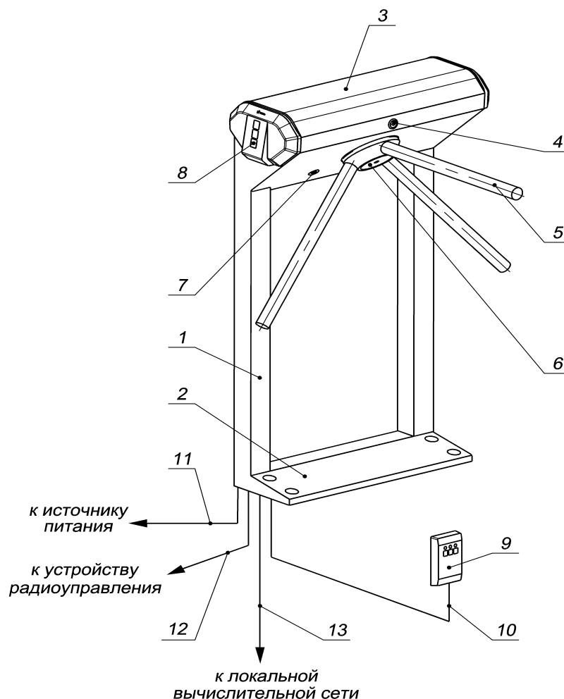
Рисунок 1 – Устройство ЭП:
