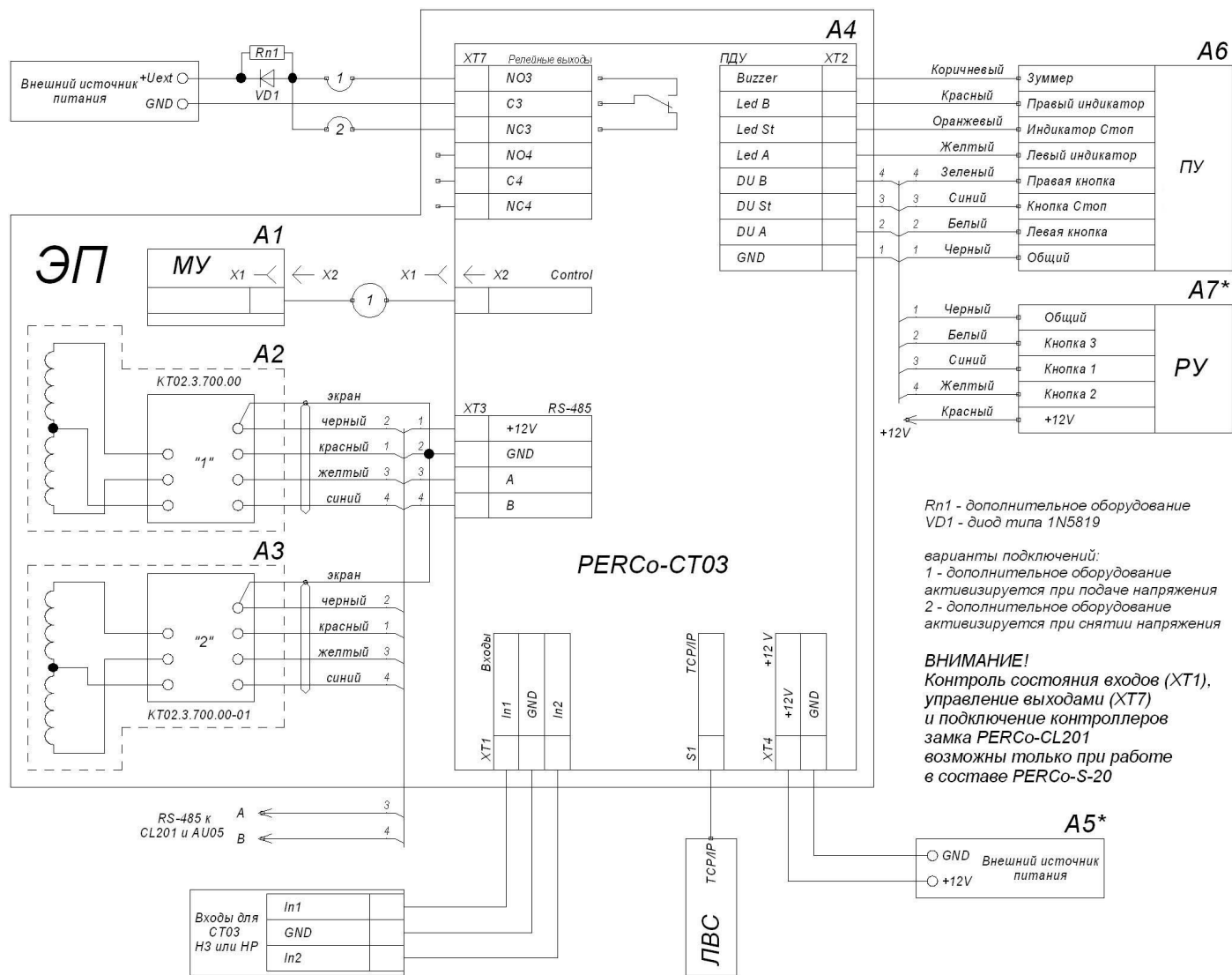
Рисунок А.1 — Схема подключения ЭП и дополнительного оборудования*
