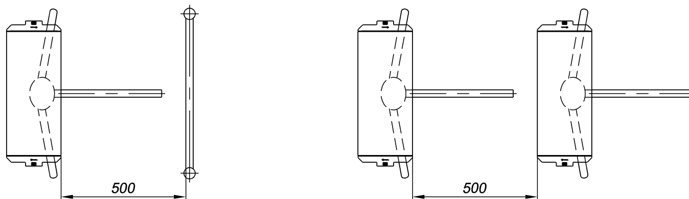
Рисунок 5 — Рекомендации по организации зоны прохода
